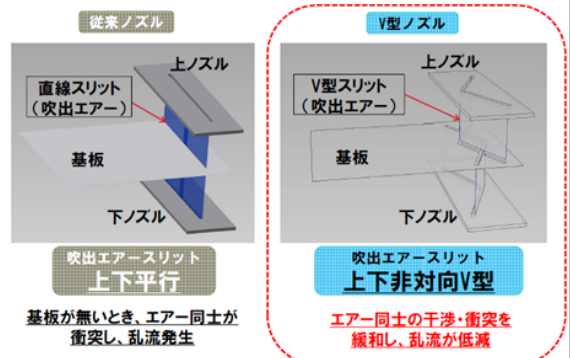
【従来ノズル】と【V型ノズル】の構造
